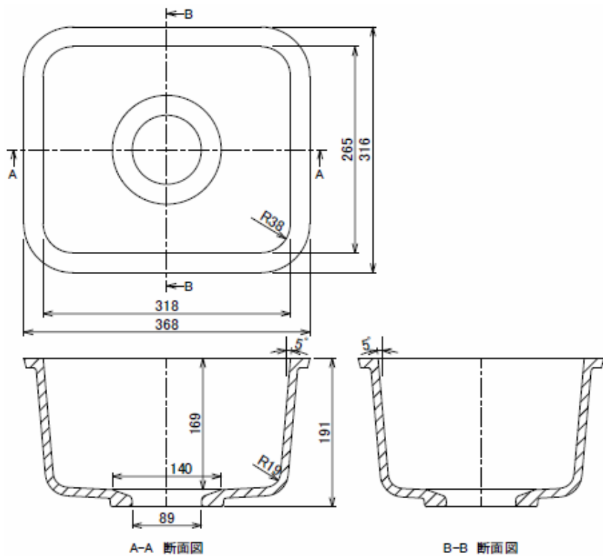
A-A 断面図
